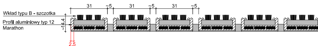
UNIMAT 12 B_M PRZEKRÓJ
