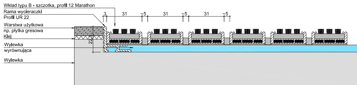
UNIMAT 12 B_M + UR 22
