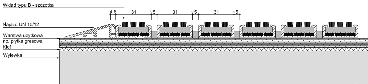
UNIMAT 12 B_M + UN 10/12
