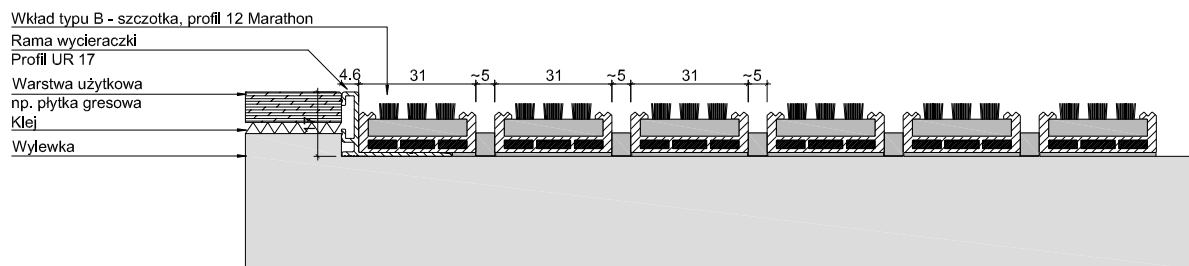
UNIMAT 12 B_M + UR 17
