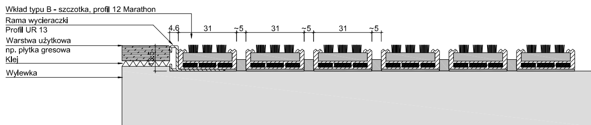
UNIMAT 12 B_M + UR 13
