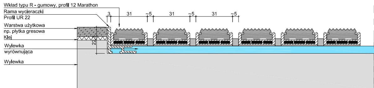
UNIMAT 12 R_M + UR 22
