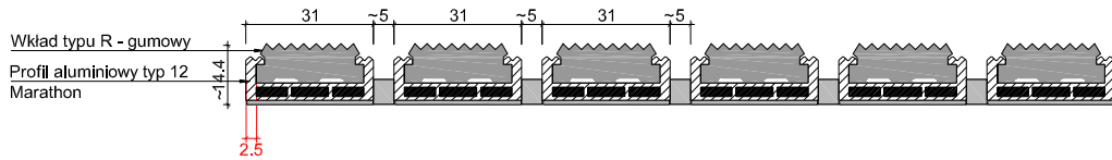
UNIMAT 12 R_M PRZEKRÓJ
