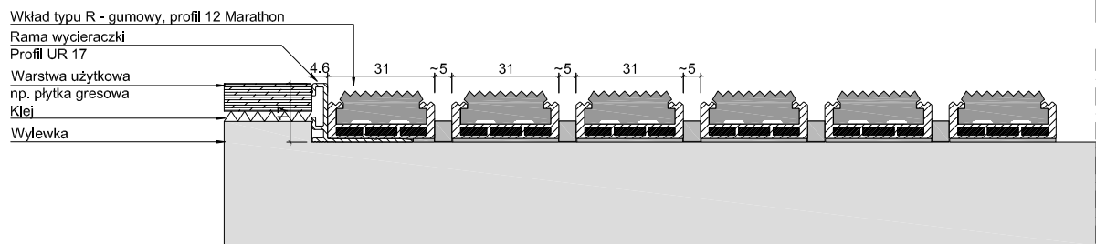
UNIMAT 12 R_M + UR 17
