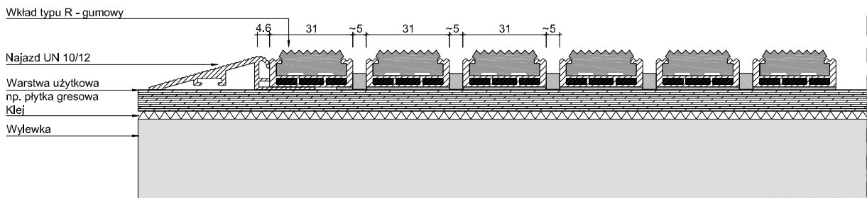
UNIMAT R_M + UN 10/12
