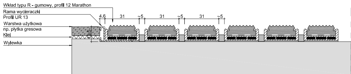
UNIMAT 12 R_M + UR 13
