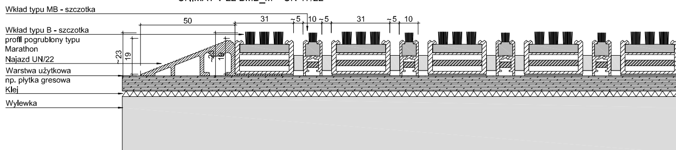
UNIMAT V 22 BMB_M + UN 17/22
