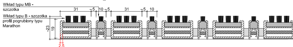
UNIMAT V 22 BMB_M PRZEKRÓJ
