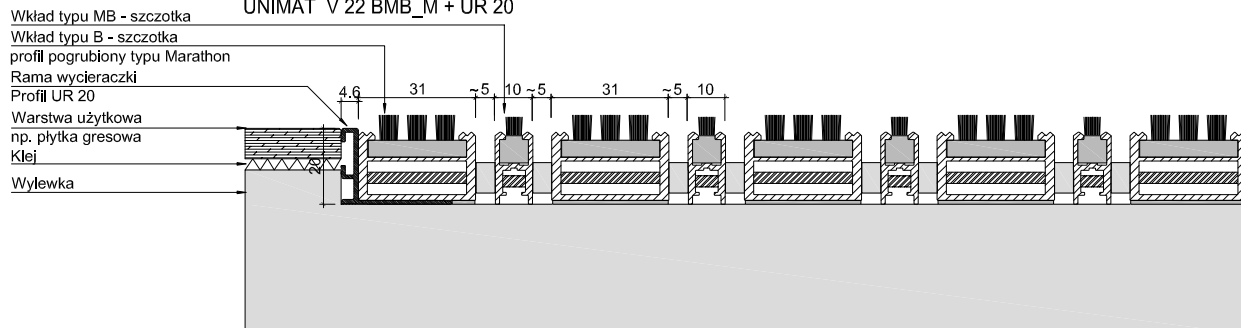
UNIMAT V 22 BMB_M + UR 20
