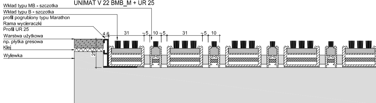
UNIMAT V 22 BMB_M + UR 25
