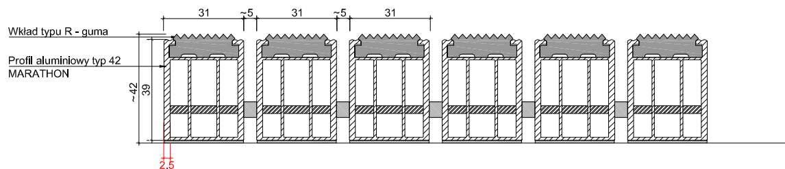
UNIMAT 42 B_M PRZEKRÓJ
