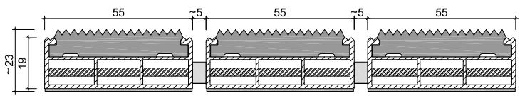
UNIMAT 22 R_P Prestige PRZEKRÓJ
