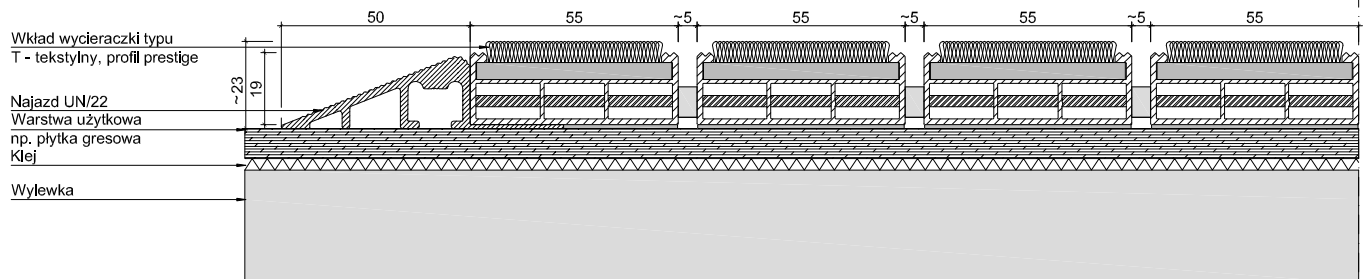
UNIMAT V 22 T_P + UN 17/22
