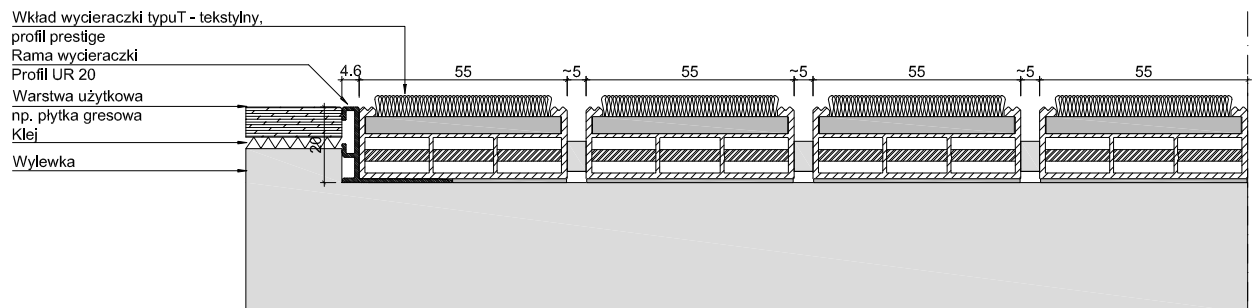
UNIMAT V 22 T_P + UR 20
