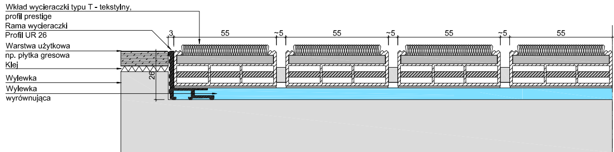
UNIMAT V 22 T_P + UR 26
