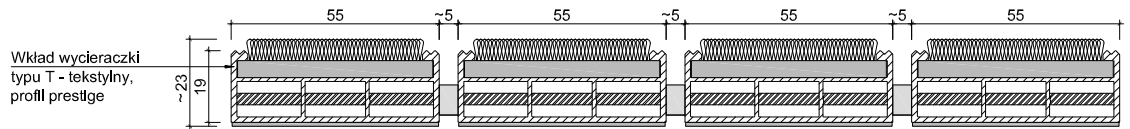
UNIMAT V 22 T_P Prestige PRZEKRÓJ
