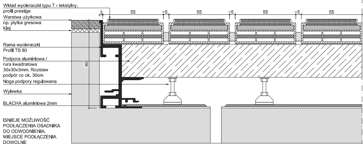
UNIMAT V 22 T_P + TS 80
