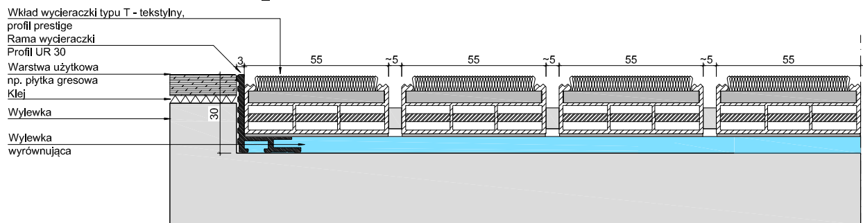
UNIMAT V 22 T_P + UR 30
