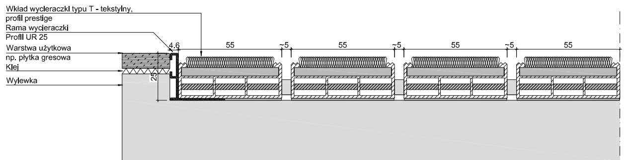
UNIMAT V 22 T_P + UR 25
