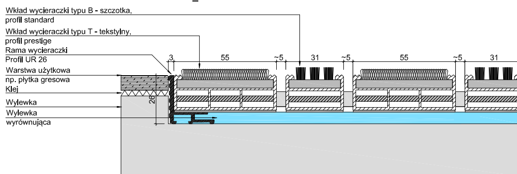
UNIMAT V 22 TB_P + UR 26
