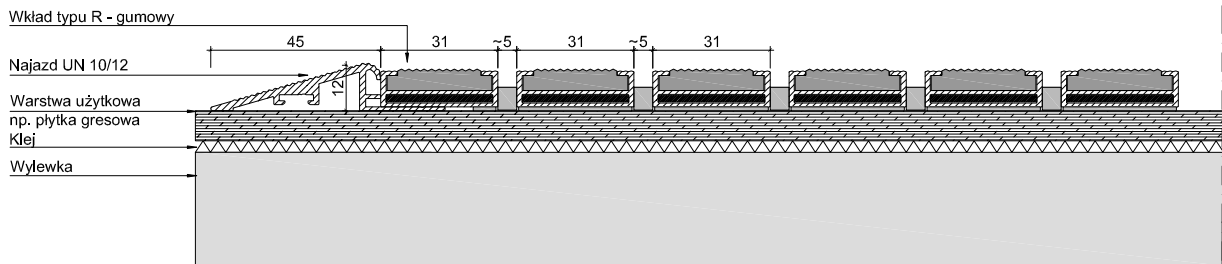
UNIMAT 10 R + UN 10/12
