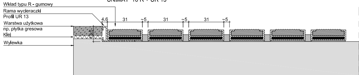
UNIMAT 10 R + UR 13
