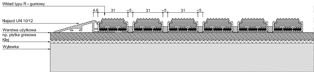
UNIMAT 12 R + UN 10/12
