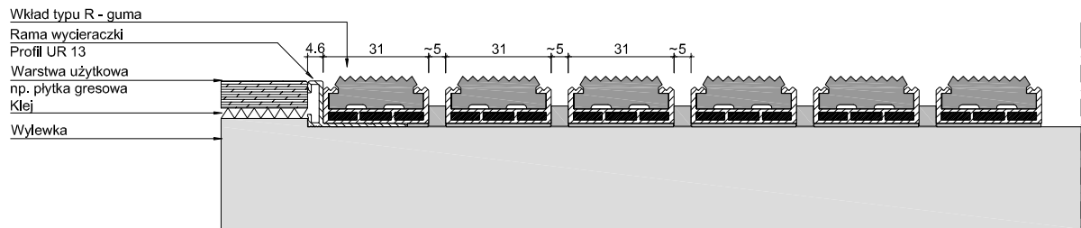
UNIMAT 12 R + UR 13
