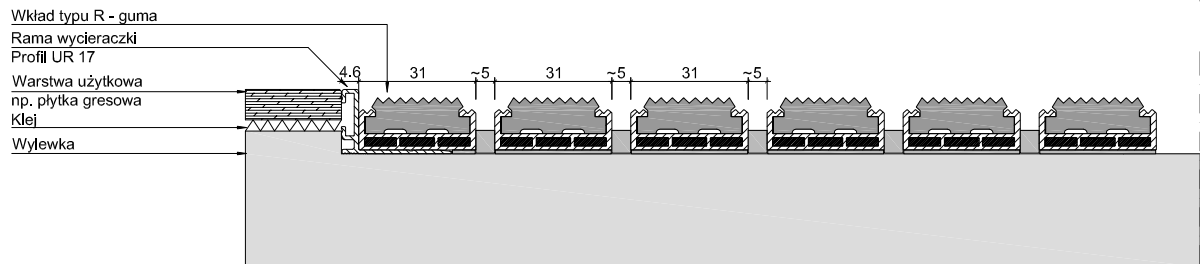
UNIMAT 12 R + UR 17
