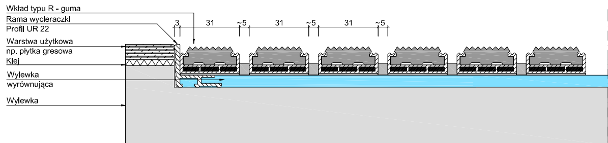
UNIMAT 12 R + UR 22
