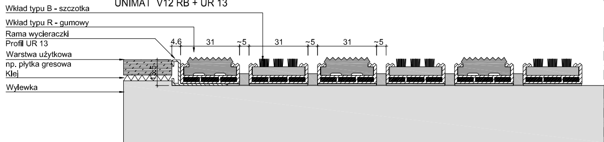
UNIMAT V12 RB + UR 13
