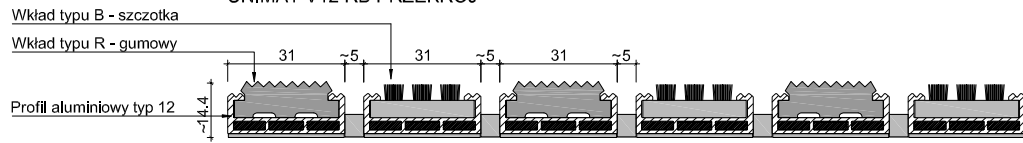
UNIMAT V12 RB PRZEKRÓJ
