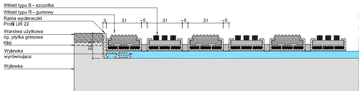
UNIMAT V12 RB + UR 22
