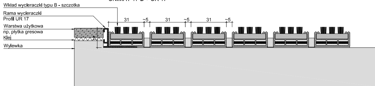
UNIMAT 17 B + UR 17
