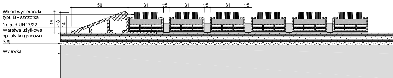
UNIMAT 17 B+ UN 17/22
