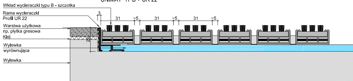
UNIMAT 17 B + UR 22
