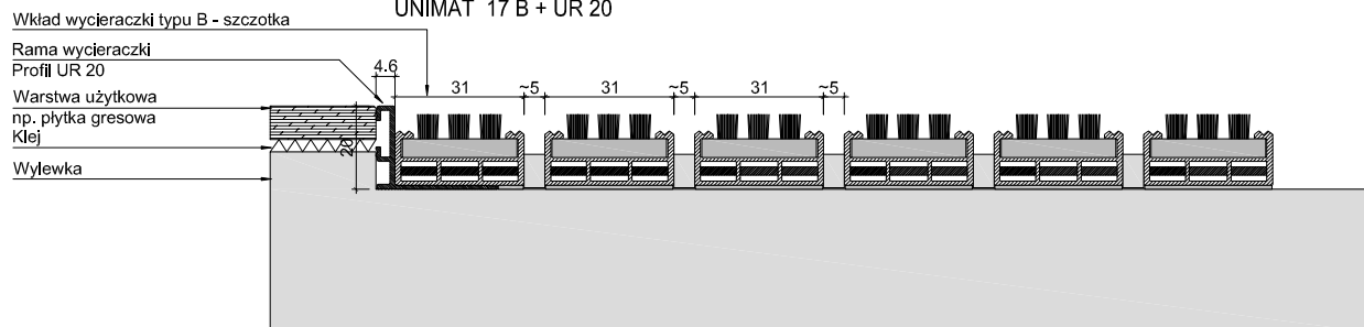
UNIMAT 17 B + UR 20
