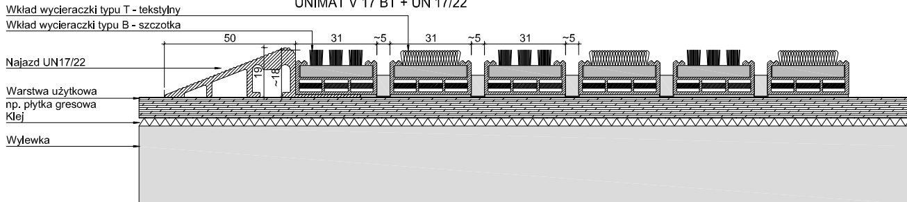
UNIMAT V 17 BT + UN 17/22
