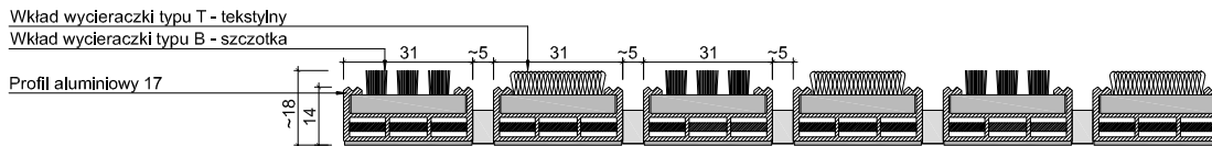
UNIMAT V 17 BT - PRZEKRÓJ
