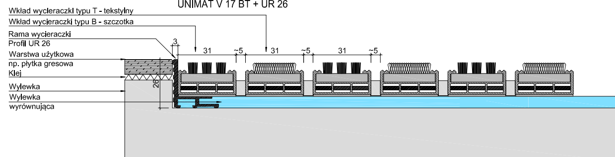
UNIMAT V 17 BT + UR 26
