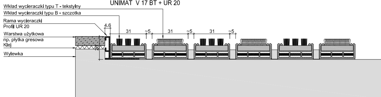
UNIMAT V 17 BT + UR 22
