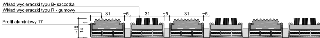
UNIMAT V 17 RB - PRZEKRÓJ
