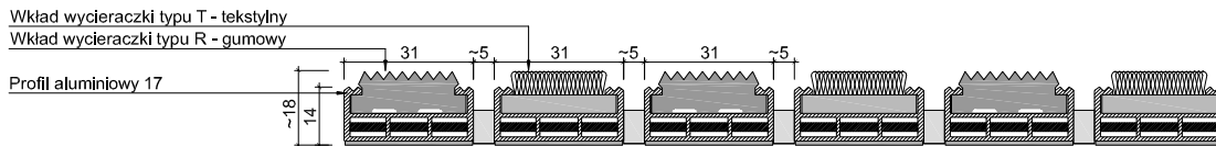
UNIMAT V 17 RT - PRZEKRÓJ
