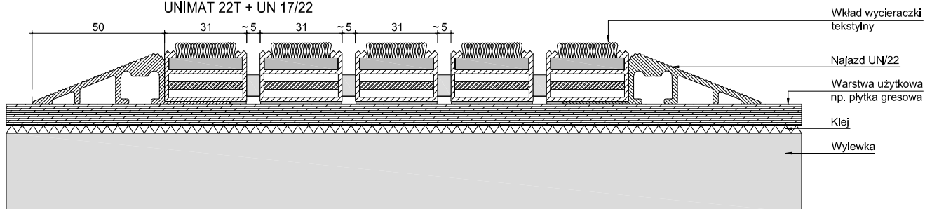
UNIMAT 22T + UN 17/22
