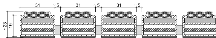
UNIMAT 22T PRZEKRÓJ
