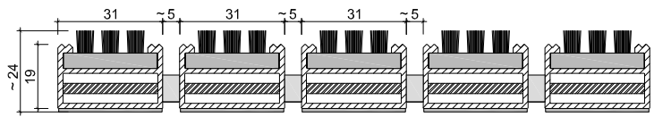
UNIMAT 22B PRZĘKRÓJ
