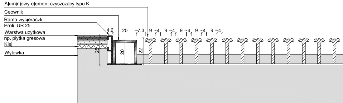
UNIMAT 22 K + UR 25
