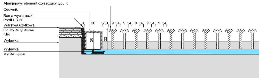
UNIMAT 22K + UR 30
