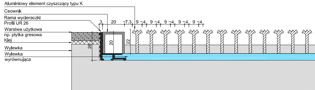
UNIMAT 22 K + UR 26
