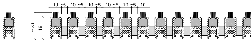
UNIMAT 22MB PRZEKRÓJ
