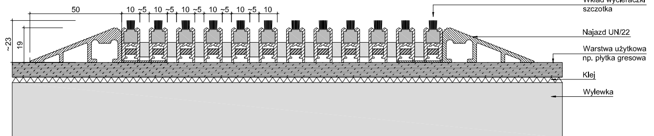
UNIMAT 22 MB + UN 17/22
