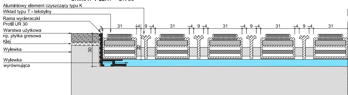
UNIMAT V 22KT + UR 30
