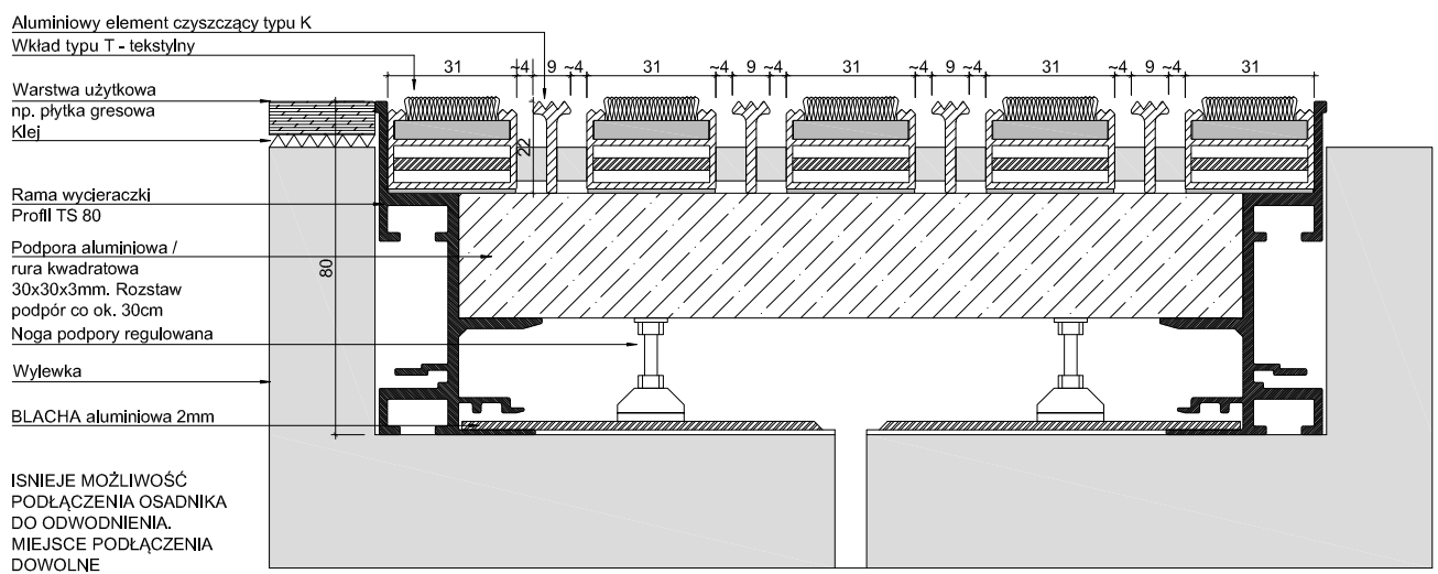
UNIMAT V 22KT + TS 80
