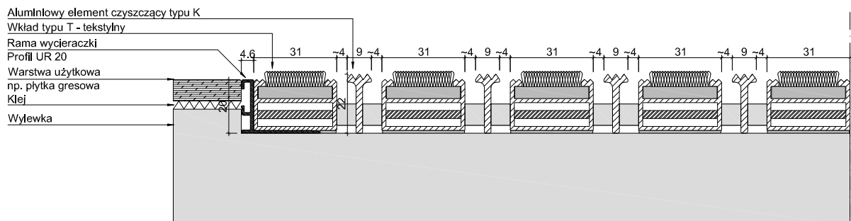
UNIMAT V 22 KT + UR 20
