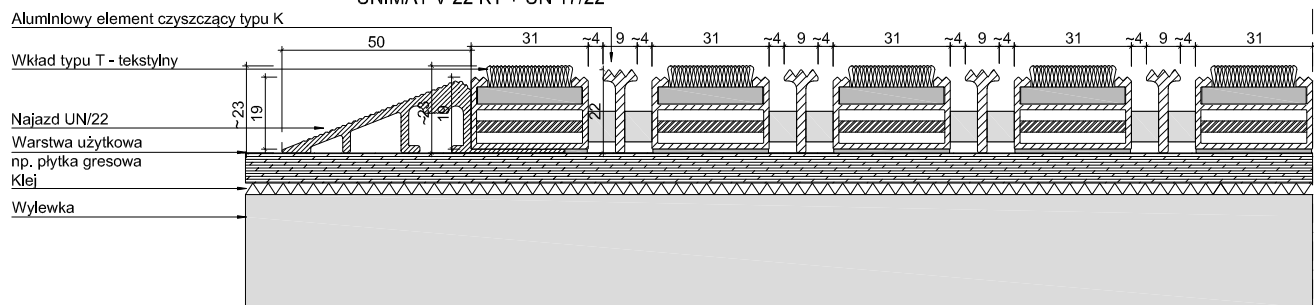
UNIMAT V 22 KT + UN 17/22
