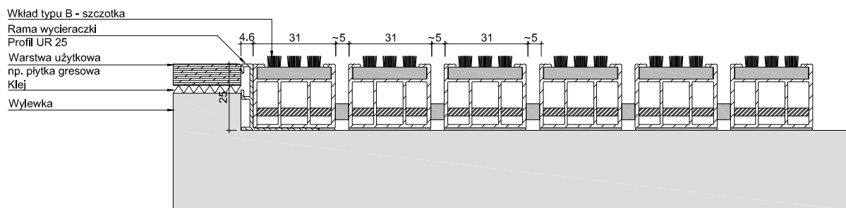
UNIMAT 27 B + UR 25
