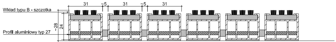
UNIMAT 27 B PRZEKRÓJ
