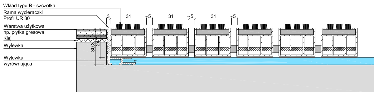
UNIMAT 27 B + UR 30
