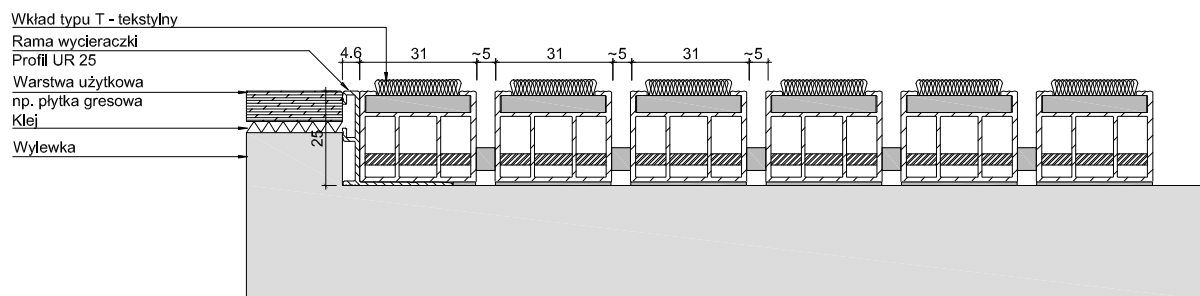
UNIMAT 27 T + UR 25
