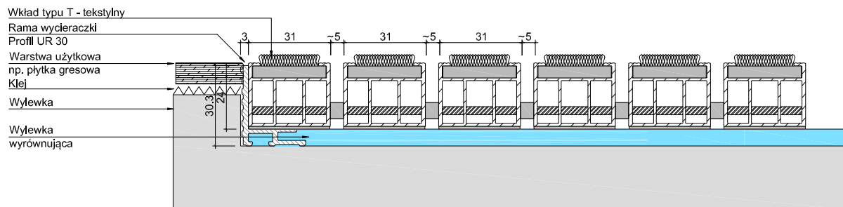
UNIMAT 27 T + UR 30
