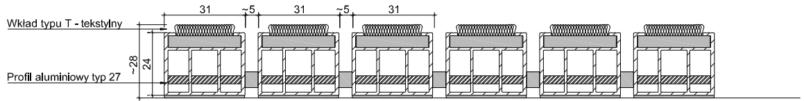
UNIMAT 27 T PRZEKRÓJ
