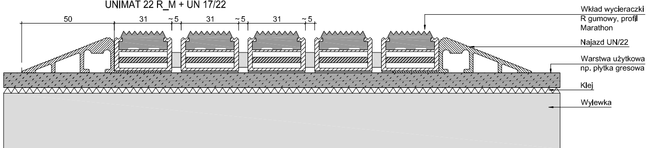
UNIMAT 22 R_M + UN 17/22
