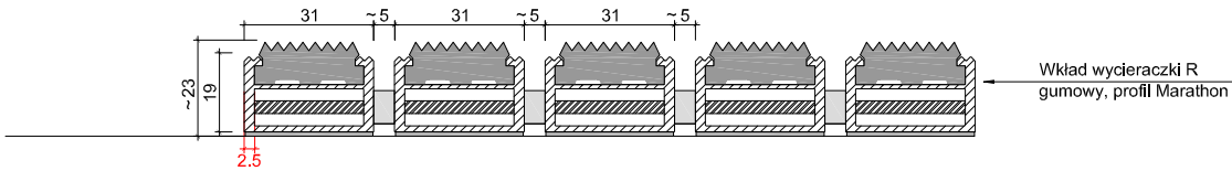
UNIMAT 22 R_M PRZEKRÓJ
